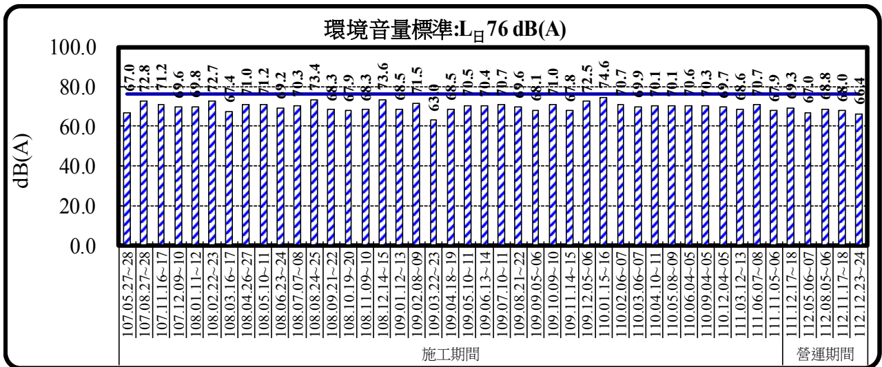
圖 2.2-1 歷次六合路(基地旁)噪音 L_{\text{日}} 監測結果分析圖
