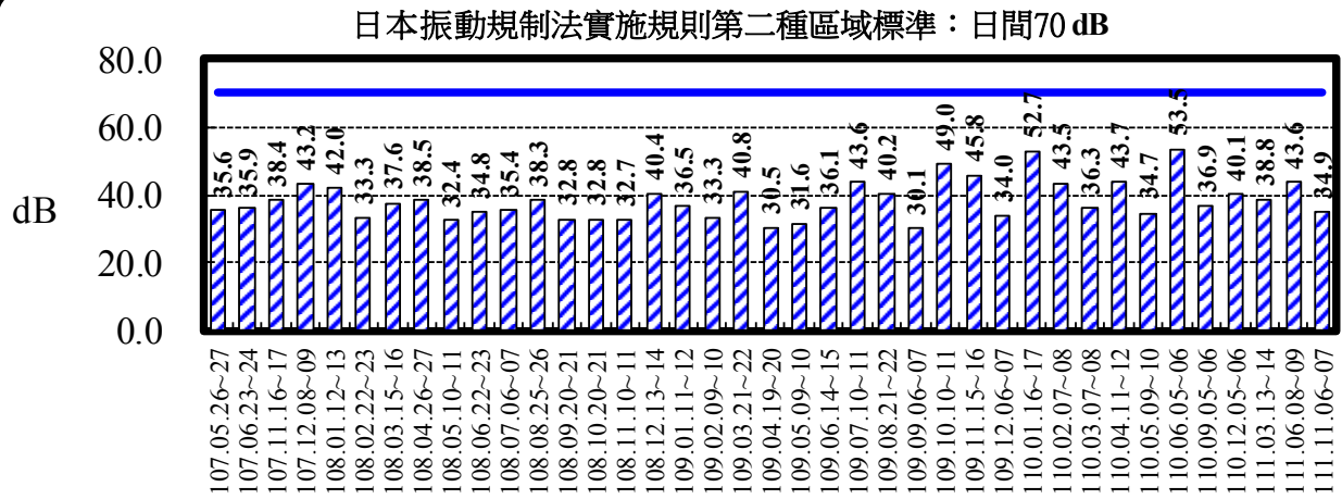
圖 2.2-17 歷次 工區周界 振動監測結果(日間)分析圖
