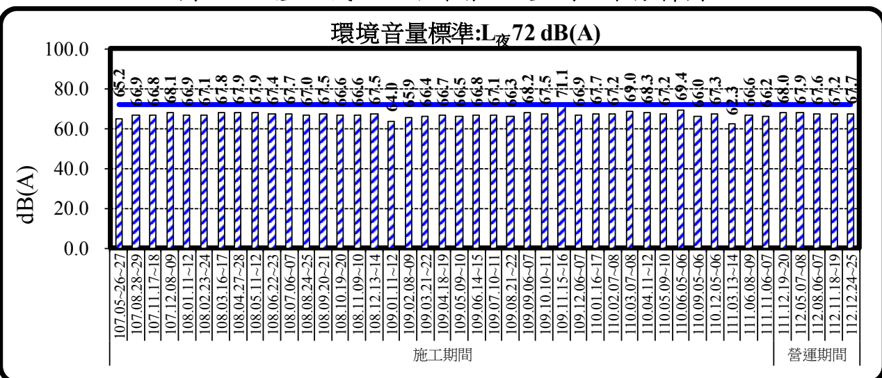
圖 2.2-6 歷次民族二路噪音 L_{\text{夜}} 監測結果分析圖
