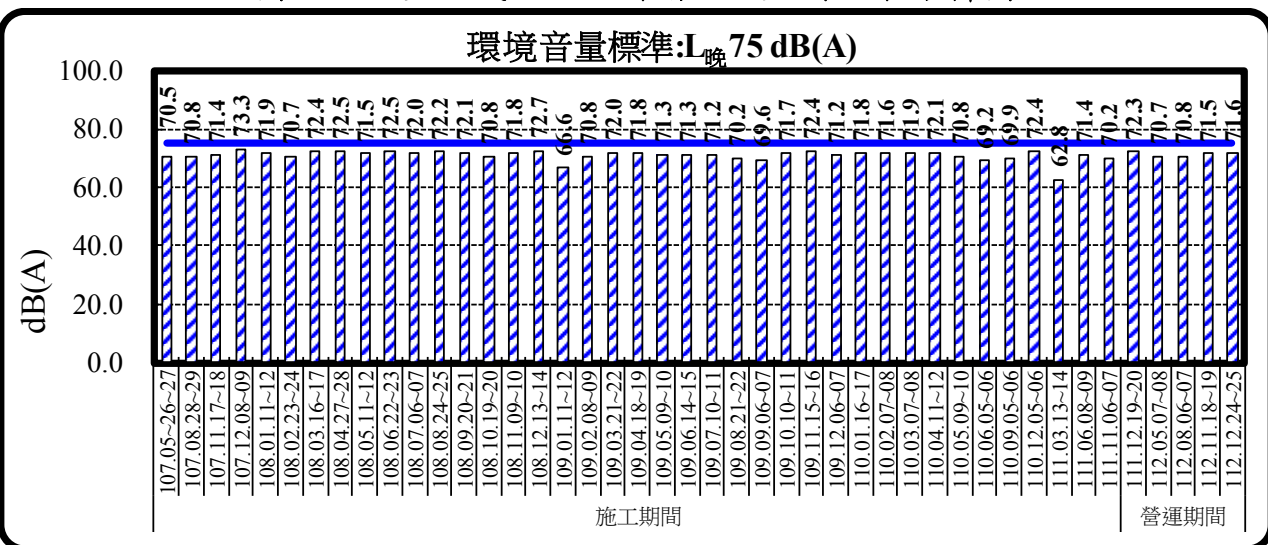
圖 2.2-5 歷次民族二路噪音 L_{\text{晚}} 監測結果分析圖
