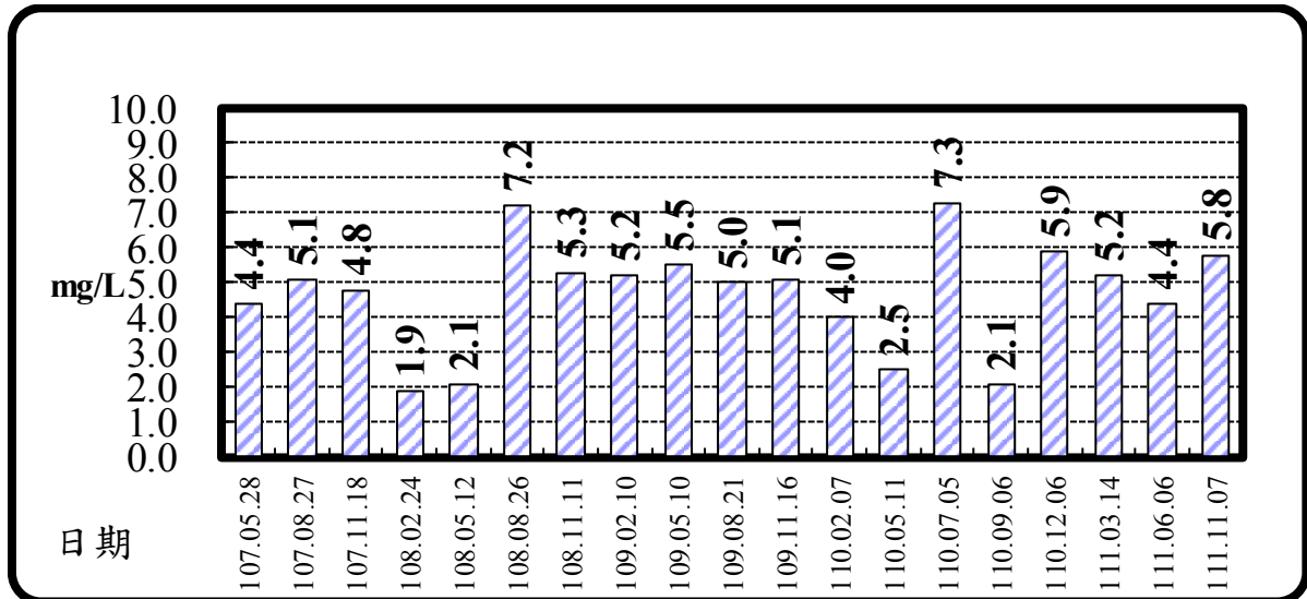
圖 2.4-3 放流水溶氧量監測結果
