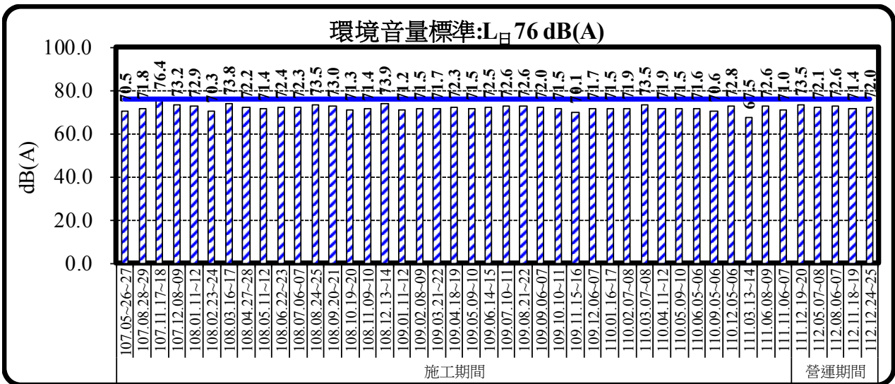
圖 2.2-4 歷次民族二路噪音 L_{\text{日}} 監測結果分析圖
