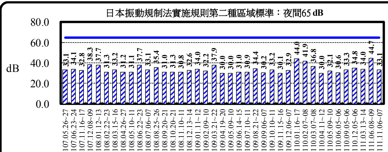
圖 2.2-18 歷次 工區周界 振動監測結果(夜間)分析圖
