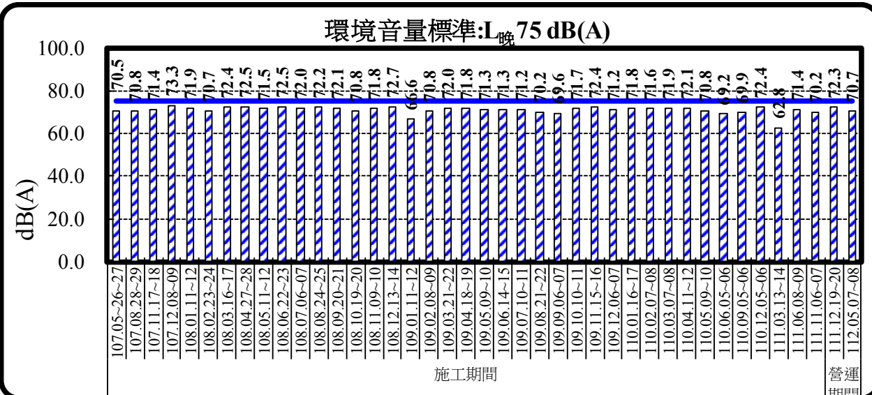
圖 2.2-5 歷次民族二路噪音 L_{\text{晚}} 監測結果分析圖
