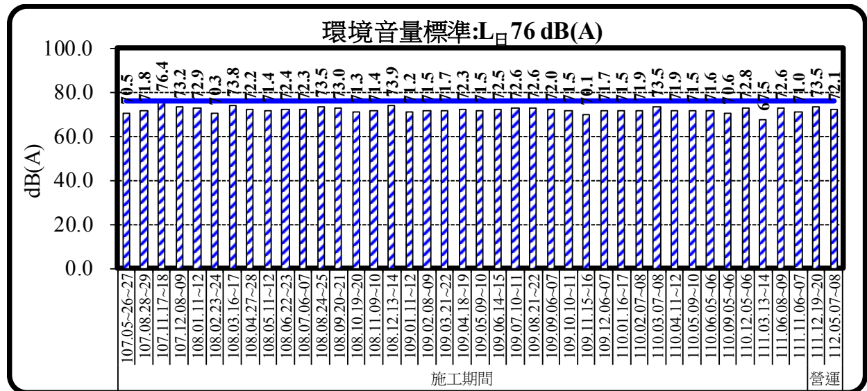
圖 2.2-4 歷次民族二路噪音 L_{\text{日}} 監測結果分析圖
