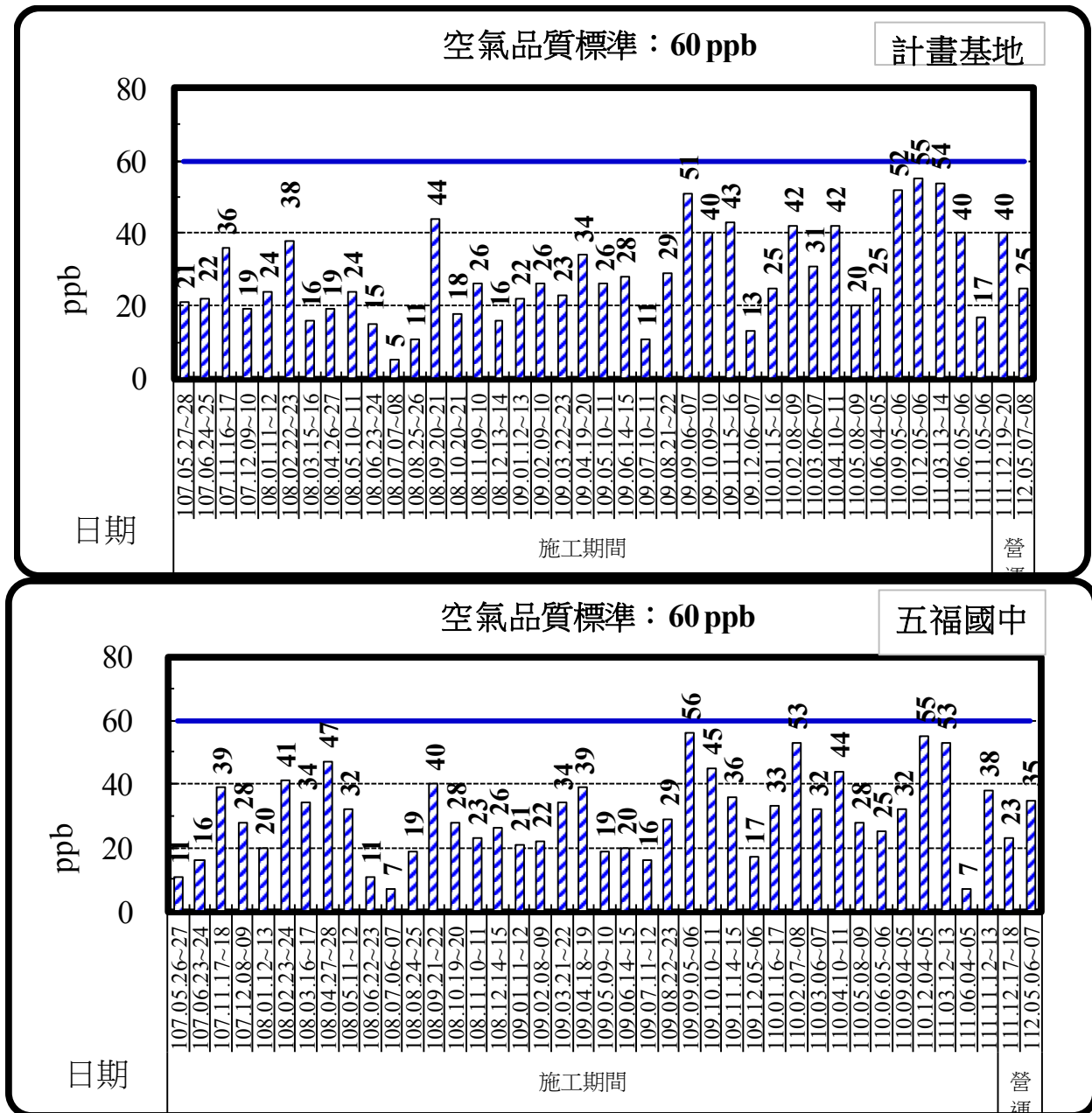
圖 2.1-10 歷次空氣品質 O 3 最大八小時平均值
